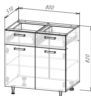
Корпус: ШН2Я800(490) (ШхВхГ) 800х820х510 мм Фасад: ЛДСП ФАСАД РИО NEW ШН2Я800
