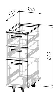
Корпус: ШНЗЯ300(490) (ШхВхГ) 300х820х510 мм Фасад: ЛДСП ФАСАД РИО NEW ШНЗЯ300
