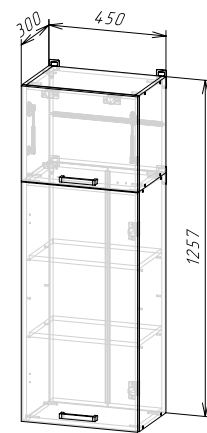
Корпус: ШВ450/1260 (ШхВхГ) 450x1257x300 мм Фасад: ЛДСП ФАСАД РИО NEW ШВ450/1260
