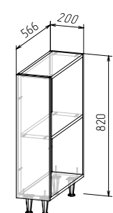
Корпус: ТР 820 (БЕЗ СТОЛЕШНИЦЫ) (ШхВхГ) 200х820х566 мм
