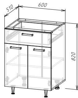
Корпус: ШН1Я600/ШН1Д1Я600(490) (ШхВхГ) 600х820х510 мм Фасад: ЛДСП ФАСАД РИО NEW ШН1Я600
