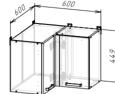
Корпус: ШВУП600/450 (ШхВхГ) 600x449x600 мм Фасад: ЛДСП ФАСАД РИО NEW ШВУП600/450
