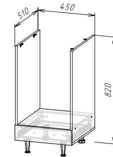
Корпус: ШНВТ450(490) (ШхВхГ) 450х820х510 мм Фасад: ЛДСП ФАСАД РИО NEW ШНВТ450
