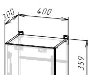
Корпус: ШВГ400/360 (ШхВхГ) 400х359х300 мм Фасад: ЛДСП ФАСАД РИО NEW ШВГ400/360 / ШВГА 400/360
