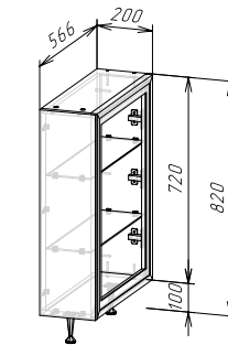
Корпус: ШНТД200 (ШхВхГ) 200х820х566 мм Фасад: ЛДСП ФАСАД РИО NEW ШВТД200/ШНТД200
