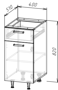
Корпус: ШН1Я400(490) (ШхВхГ) 400х820х510 мм Фасад: ЛДСП ФАСАД РИО NEW ШН1Я400
