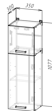
Корпус: ШВ350/1080 (ШхВхГ) 350x1077x300 мм Фасад: ЛДСП ФАСАД РИО NEW ШВ350/1080
