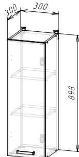
Корпус: ШВ300/900 / ШВС300/900 (ШхВхГ) 300х898х300 мм Фасад: ЛДСП ФАСАД РИО NEW ШВ300/900
