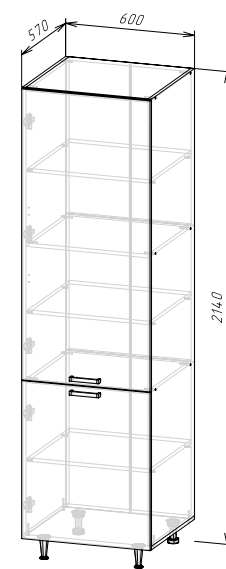
Корпус: ШП600/ШП600-1/ШП600-2 (ШхВхГ) 600x2140x570 мм Фасад: ЛДСП ФАСАД РИО NEW ШП600-2
