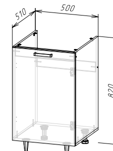
Корпус: ШНМ500(490) (ШхВхГ) 500х820х510 мм Фасад: ЛДСП ФАСАД РИО NEW ШН500/ШН500/ШНМ500
