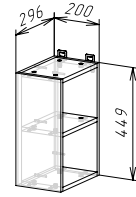
Корпус: ШВТ200/450 (ШхВхГ) 200х449х300 мм Фасад: ЛДСП ФАСАД РИО NEW ШВТ200/450
