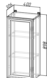
Корпус: ШВ-П400/900 (ШхВхГ) 400х898х306 мм Фасад: РАМКА AGT ШВ400/900
