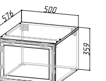
Корпус: ШВГА-П500/360 (ШхВхГ) 500х359х576 мм Фасад: РАМКА AGT ШВГ/ ШВГА 500/360
