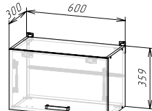
Корпус: ШВГ600/360 / ШВГС600/360 (ШхВхГ) 600х359х300 мм Фасад: ЛДСП ФАСАД РИО NEW ШВГ600/360 / ШВГА 600/360
