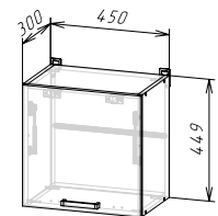
Корпус: ШВГ450/450 (ШхВхГ) 450х449х300 мм Фасад: ЛДСП ФАСАД РИО NEW ШВГ450/450 / ШВГА450/450
