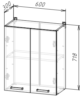
Корпус: ШВ600/ШВС600/ ШВ1Д600/ШВС1Д600 (ШхВхГ) 600х718х300 мм Фасад: ЛДСП ФАСАД РИО NEW ШВ600/ШН600/ШНМ600
