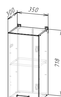
Корпус: ШВ350 (ШхВхГ) 350х718х300 мм Фасад: ЛДСП ФАСАД РИО NEW ШВ350/ШН350
