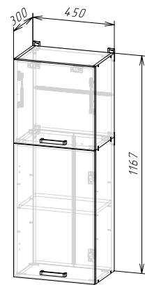
Корпус: ШВ450/1170 (ШхВхГ) 450x1167x300 мм Фасад: ЛДСП ФАСАД РИО NEW ШВ450/1170
