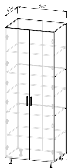
Корпус: ШП800/ШПС800/ ШП800-1 (ШхВхГ) 800x2140x570 мм Фасад: ЛДСП ФАСАД РИО NEW ШП800-1
