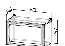
Корпус: ШВГ-П600/360 (ШхВхГ) 600х359х306 мм Фасад: РАМКА AGT ШВГ/ ШВГА 600/360
