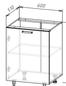
Корпус: ШН600/ШН1Д600(490) (ШхВхГ) 600х820х510 мм Фасад: ЛДСП ФАСАД РИО NEW ШН1Д600/ШН1Д600/ШНМ1Д600
