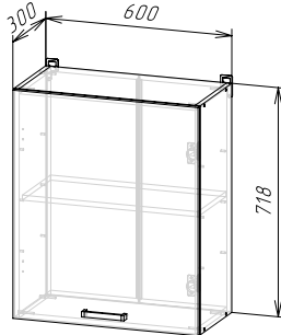
Корпус: ШВ600/ШВС600/ ШВ1Д600/ШВС1Д600 (ШхВхГ) 600х718х300 мм Фасад: ЛДСП ФАСАД РИО NEW ШВ1Д600/ШН1Д600/ШНМ1Д600
