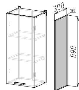
ЛДСП ФАСАД РИО NEW БФП (898х300) (ШхВхГ) 898х300х16 мм
