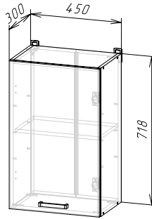
Корпус: ШВ450/ШВС450 (ШхВхГ) 450х718х300 мм Фасад: ЛДСП ФАСАД РИО NEW ШВ450/ШН450
