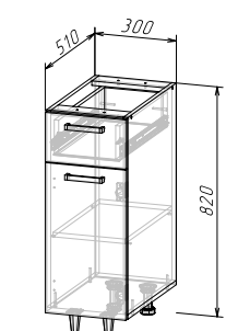
Корпус: ШН1Я300(490) (ШхВхГ) 300х820х510 мм Фасад: ЛДСП ФАСАД РИО NEW ШН1Я300
