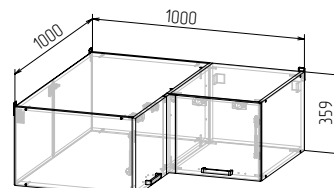
Корпус: ШВГАУП1000 (ШхВхГ) 1000x359x1000 мм Фасад: ЛДСП ФАСАД РИО NEW ШВГ800/360 / ШВГА 800/360
