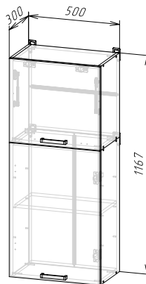
Корпус: ШВ500/1170 (ШхВхГ) 500x1167x300 мм Фасад: ЛДСП ФАСАД РИО NEW ШВ500/1170
