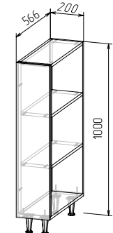
Корпус: ТР 1000 (ШхВхГ) 200х1000х566 мм
