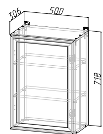
Корпус: ШВ-П500 (ШхВхГ) 500х718х306 мм Фасад: РАМКА AGT ШВ500
