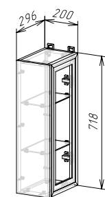
Корпус: ШВТД200 (ШхВхГ) 200х718х300 мм Фасад: ЛДСП ФАСАД РИО NEW ШВТД200/ШНТД200
