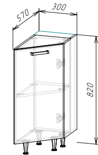
Корпус: ШНТД300 (ШхВхГ) 300х820х570 мм Фасад: ЛДСП ФАСАД РИО NEW ШНТД300
