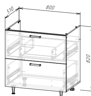
Корпус: ШНМ2ЯГ800(490) (ШхВхГ) 800х820х510 мм Фасад: ЛДСП ФАСАД РИО NEW ШНМ2ЯГ800
