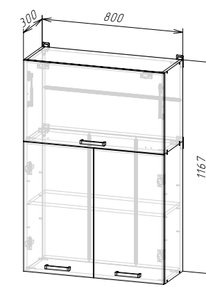
Корпус: ШВ800/1170 (ШхВхГ) 800x1167x300 мм Фасад: ЛДСП ФАСАД РИО NEW ШВ800/1170
