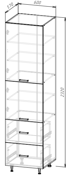
Корпус: ШПВ2Я600/ШПВ2Я600-1/ ШПВ2Я600-2 (ШхВхГ) 600х2320х570 мм Фасад: ЛДСП ФАСАД РИО NEW ШПВ2Я600-1
