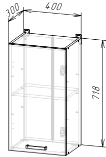
Корпус: ШВ400/ШВС400 (ШхВхГ) 400х718х300 мм Фасад: ЛДСП ФАСАД РИО NEW ШВ400/ШН400
