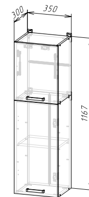
Корпус: ШВ350/1170 (ШхВхГ) 350x1167x300 мм Фасад: ЛДСП ФАСАД РИО NEW ШВ350/1170
