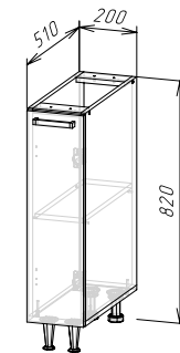
Корпус: ШН200(490) (ШхВхГ) 200х820х510 мм Фасад: ЛДСП ФАСАД РИО NEW ШН200/ШН200
