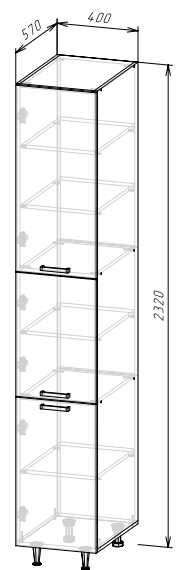
Корпус: ШПВ400/ШПВ400-1 (ШхВхГ) 400х2320х570 мм Фасад: ЛДСП ФАСАД РИО NEW ШПВ400
