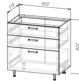
Корпус: ШНЗЯ800(490) (ШхВхГ) 800х820х510 мм Фасад: ЛДСП ФАСАД РИО NEW ШНЗЯ800
