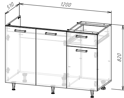
Корпус: ШН1Я1200(490) (ШхВхГ) 1200х820х510 мм Фасад: ЛДСП ФАСАД РИО NEW ШН1Я1200
