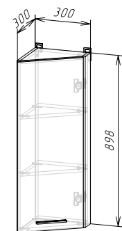
Корпус: ШВТД300/900 (ШхВхГ) 300х898х300 мм Фасад: ЛДСП ФАСАД РИО NEW ШВТД300/900
