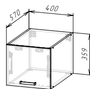
Корпус: ШВГА400/360 (ШхВхГ) 400x359x570 мм Фасад: ЛДСП ФАСАД РИО NEW ШВГ400/360 / ШВГА 400/360
