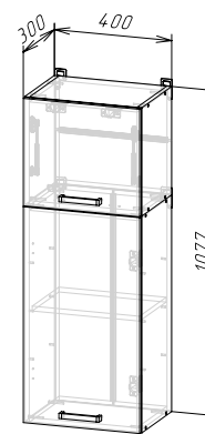
Корпус: ШВ400/1080 (ШхВхГ) 400x1077x300 мм Фасад: ЛДСП ФАСАД РИО NEW ШВ400/1080
