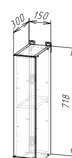
Корпус: ШВ150 (ШхВхГ) 150х718х300 мм Фасад: ЛДСП ФАСАД РИО NEW ШВ150/ШН150
