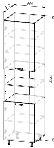
Корпус: ШПВ600/ШПВ600-1/ШПВ600-2 (ШхВхГ) 600х2320х570 мм Фасад: ЛДСП ФАСАД РИО NEW ШПВ600
