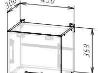
Корпус: ШВГ450/360 (ШхВхГ) 450х359х300 мм Фасад: ЛДСП ФАСАД РИО NEW ШВГ450/360 / ШВГА 450/360
