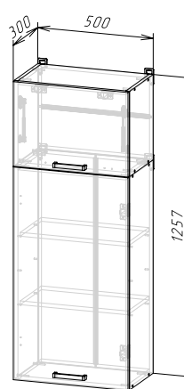
Корпус: ШВ500/1260 (ШхВхГ) 500x1257x300 мм Фасад: ЛДСП ФАСАД РИО NEW ШВ500/1260
