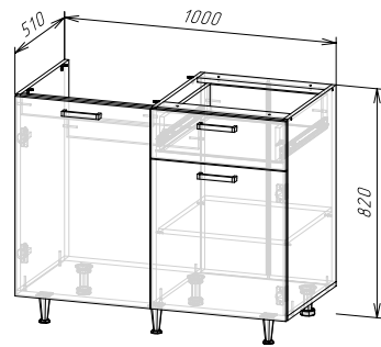
Корпус: ШН1Я1000(490) (ШхВхГ) 1000х820х510 мм Фасад: ЛДСП ФАСАД РИО NEW ШН1Я1000
