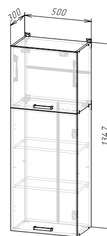
Корпус: ШВ500/1350 (ШхВхГ) 500x1347x300 мм Фасад: ЛДСП ФАСАД РИО NEW ШВ500/1350
