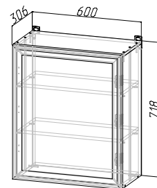
Корпус: ШВ1Д-П600 (ШхВхГ) 600х718х306 мм Фасад: РАМКА AGT ШВ1Д600
