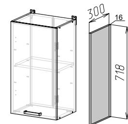
ЛДСП ФАСАД РИО NEW БФП (718х300) (ШхВхГ) 718х300х16 мм
