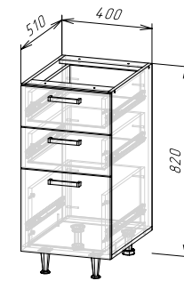
Корпус: ШНЗЯ400(490) (ШхВхГ) 400х820х510 мм Фасад: ЛДСП ФАСАД РИО NEW ШНЗЯ400
