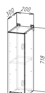
Корпус: ШВ200 (ШхВхГ) 200х718х300 мм Фасад: ЛДСП ФАСАД РИО NEW ШВ200/ШН200
