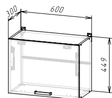
Корпус: ШВГ600/450 (ШхВхГ) 600х449х300 мм Фасад: ЛДСП ФАСАД РИО NEW ШВГ600/450
