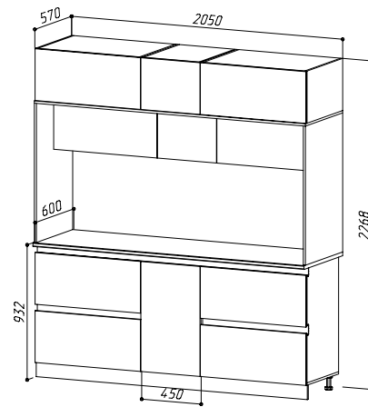
ЦЕНТРАЛЬНАЯ СЕКЦИЯ 2050 (С МЕСТОМ ПОД МП) (ШхВхГ) 2050х2268х600 мм место под МП (ШхВхГ) 450х849х533 мм
