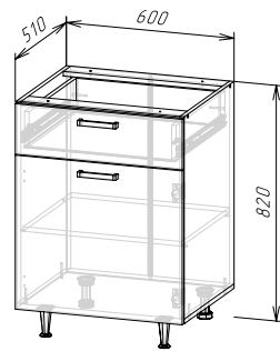
Корпус: ШН1Я600/ШН1Д1Я600(490) (ШхВхГ) 600х820х510 мм Фасад: ЛДСП ФАСАД РИО NEW ШН1Д1Я600
