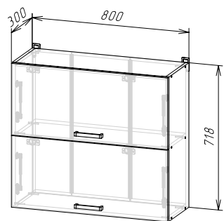
Корпус: ШВГ800/ШВГС800 (ШхВхГ) 800х718х300 мм Фасад: ЛДСП ФАСАД РИО NEW ШВГ800
