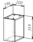
Корпус: ШВТ200/360 (ШхВхГ) 200х359х300 мм Фасад: ЛДСП ФАСАД РИО NEW ШВТ200/360
