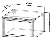
Корпус: ШВГА-П600/360 (ШхВхГ) 600х359х576 мм Фасад: РАМКА AGT ШВГ/ ШВГА 600/360
