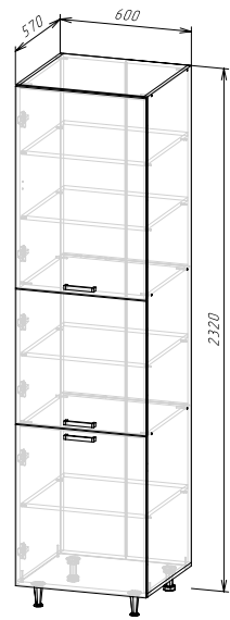
Корпус: ШПВ600/ШПВ600-1/ШПВ600-2 (ШхВхГ) 600х2320х570 мм Фасад: ЛДСП ФАСАД РИО NEW ШПВ600-1
