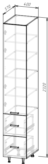
Корпус: ШПВ2Я400/ШПВ2Я400-1 (ШхВхГ) 400х2320х570 мм Фасад: ЛДСП ФАСАД РИО NEW ШПВ2Я400-1
