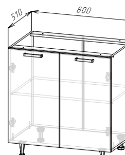
Корпус: ШН800(490) (ШхВхГ) 800х820х510 мм Фасад: ЛДСП ФАСАД РИО NEW ШН800/ШН800/ШНМ800
