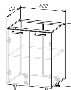
Корпус: ШН600/ШН1Д600(490) (ШхВхГ) 600х820х510 мм Фасад: ЛДСП ФАСАД РИО NEW ШН600/ШН600/ШНМ600
