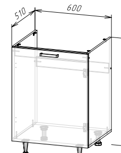
Корпус: ШНМ600/ШНМ1Д600(490) (ШхВхГ) 600х820х510 мм Фасад: ЛДСП ФАСАД РИО NEW ШН1Д600/ШН1Д600/ШНМ1Д600
