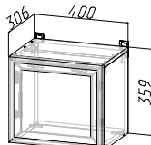
Корпус: ШВГ-П400/360 (ШхВхГ) 400х359х306 мм Фасад: РАМКА AGT ШВГ/ ШВГА 400/360
