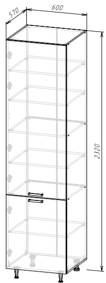
Корпус: ШПВ600/ШПВ600-1/ШПВ600-2 (ШхВхГ) 600х2320х570 мм Фасад: ЛДСП ФАСАД РИО NEW ШПВ600-2
