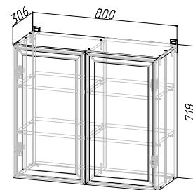
Корпус: ШВСП-П800 (ШхВхГ) 800х718х306 мм Фасад: РАМКА AGT ШВ800
