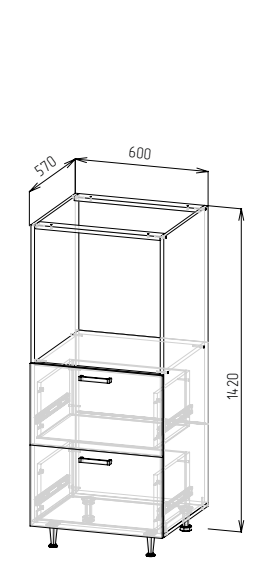
Корпус: ШПН2ЯГ (ШхВхГ) 600x1420x570 мм Фасад: ЛДСП ФАСАД РИО NEW ШН2ЯГ600
