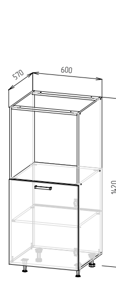
Корпус: ШПН600 (ШхВхГ) 600x1420x570 мм Фасад: ЛДСП ФАСАД РИО NEW ШВ1Д600/ШНМ1Д600/ШН1Д600
