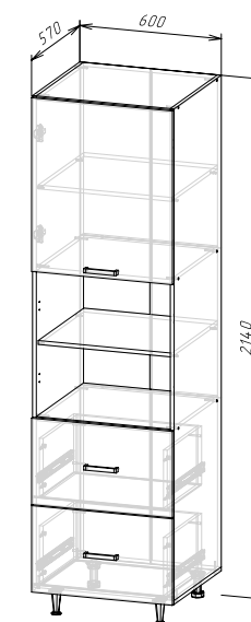
Корпус: ШП2Я600/ШП2Я600-1/ ШП2Я600-2 (ШхВхГ) 600x2140x570 мм Фасад: ЛДСП ФАСАД РИО NEW ШП2Я600
