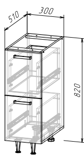
Корпус: ШН2ЯГ300(490) (ШхВхГ) 300х820х510 мм Фасад: ЛДСП ФАСАД РИО NEW ШН2ЯГ300
