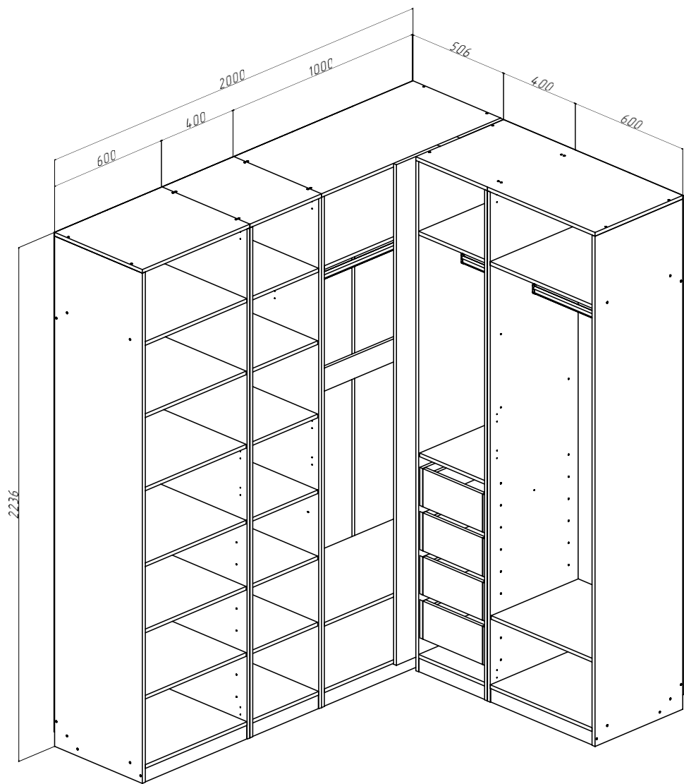
Ларго Вариант №13 (без фасадов) (ШхВхГ) 2000х2236х1506 мм
