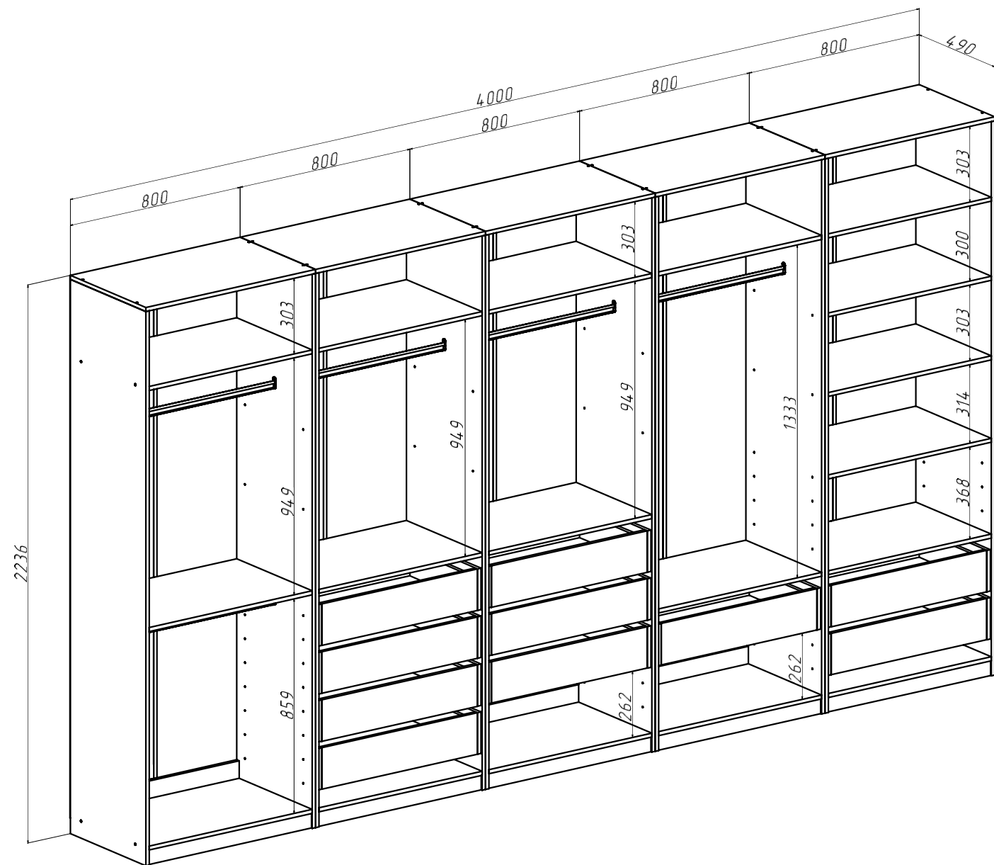
Ларго Вариант №1 (без фасадов) (ШхВхГ) 4000х2236х490 мм
