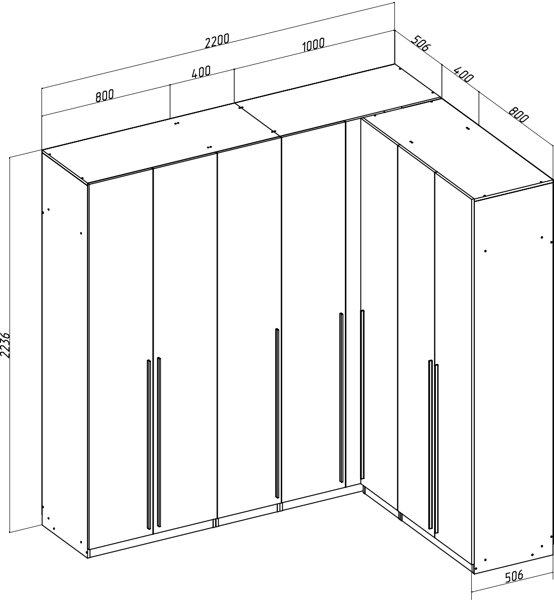
Ларго Вариант №3 (с фасадами) (ШхВхГ) 2200х2236х1706 мм
