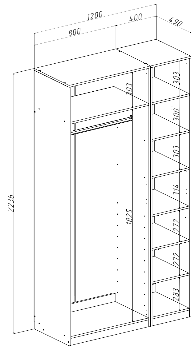
Ларго Вариант №9 (без фасадов) (ШхВхГ) 1200х2236х490 мм
