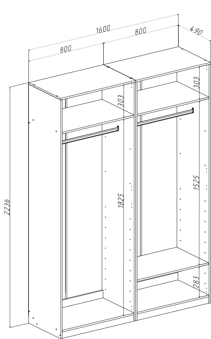
Ларго Вариант №5 (без фасадов) (ШхВхГ) 1600х2236х490 мм
