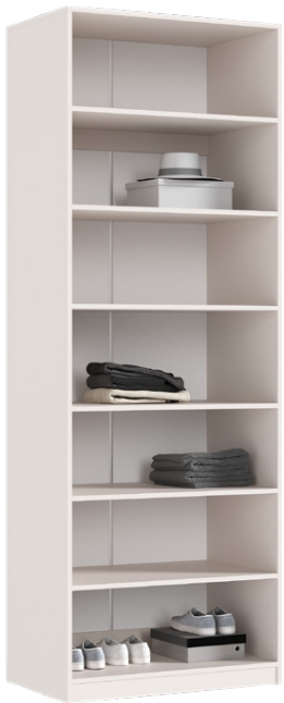
Шкаф (800) + 5 полок (ШхВхГ) 800x2236x490 мм
