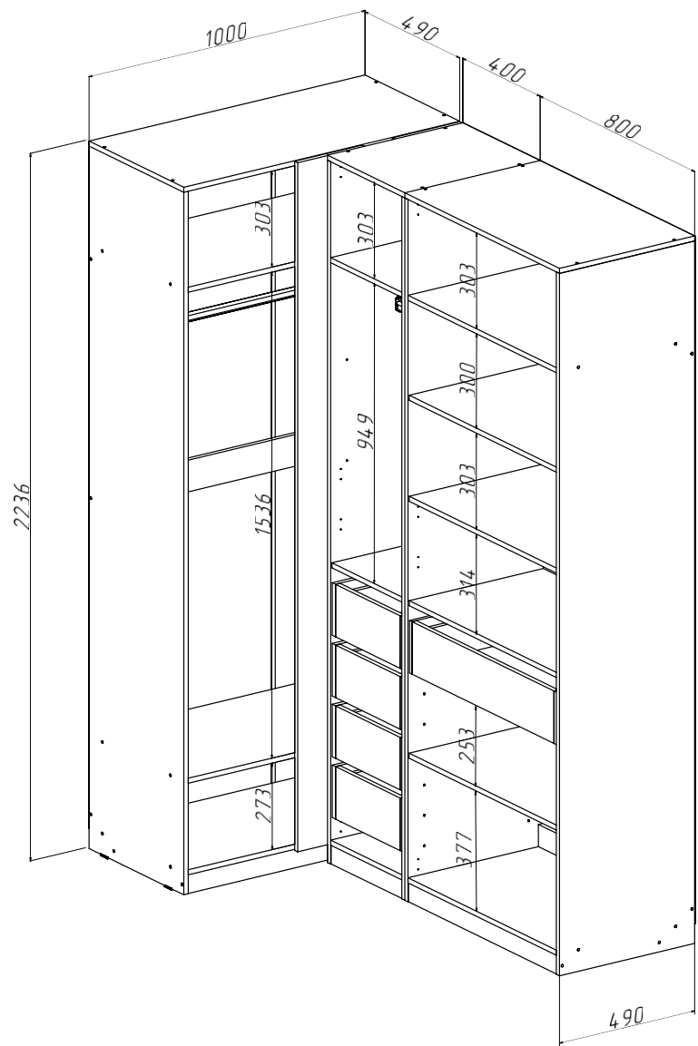
Ларго Вариант №12 (без фасадов) (ШхВхГ) 1000х2236х1690 мм
