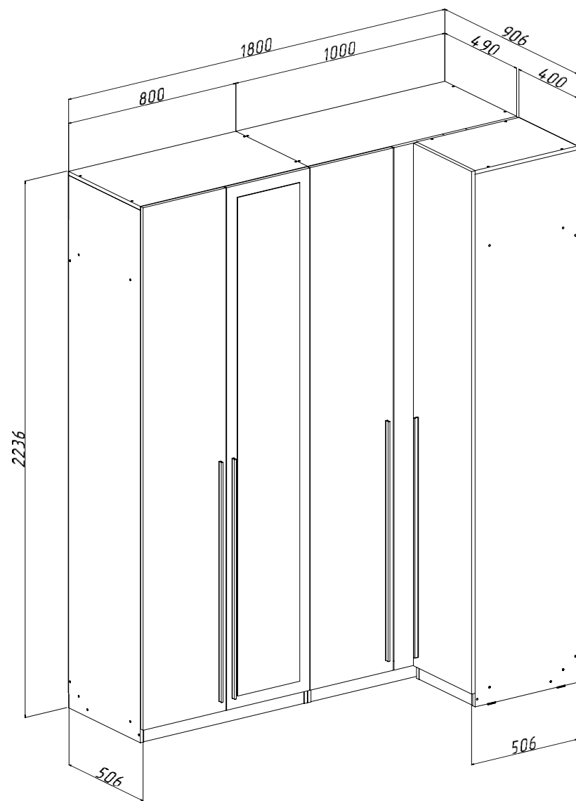
Ларго Вариант №11 (с фасадами) (ШхВхГ) 1800х2236х906 мм
