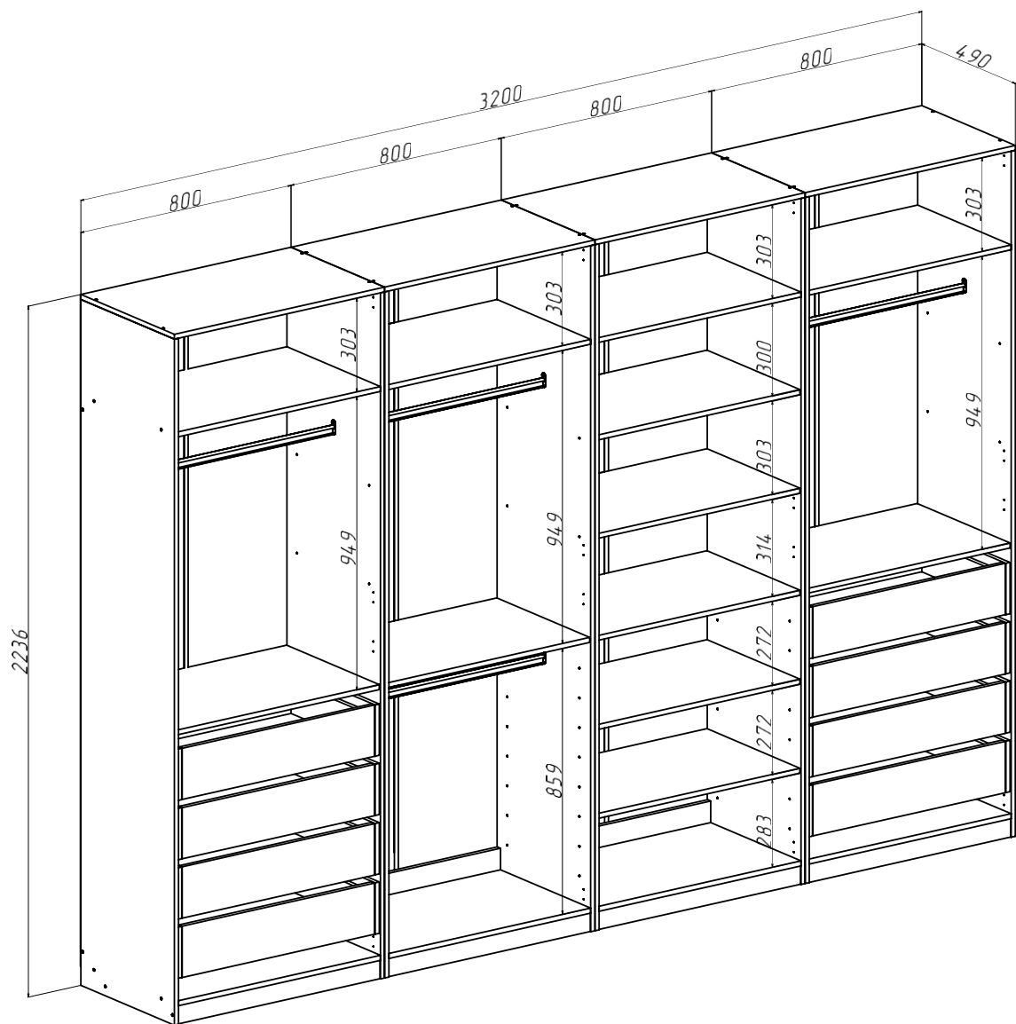
Ларго Вариант №2 (без фасадов) (ШхВхГ) 3200х2236х490 мм
