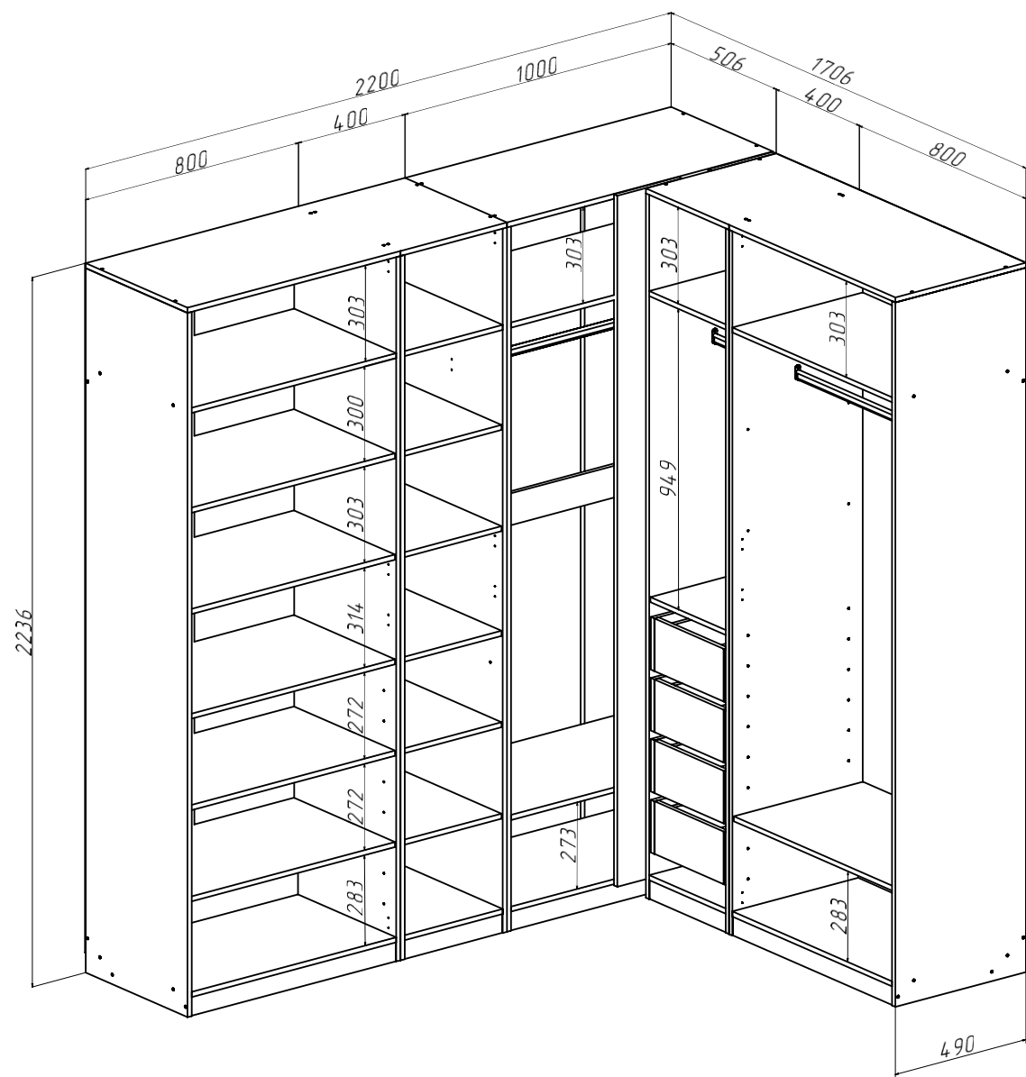
Ларго Вариант №3 (без фасадов) (ШхВхГ) 2200х2236х1706 мм
