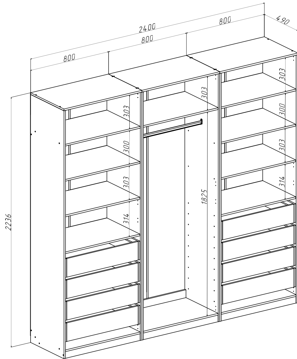
Ларго Вариант №6 (без фасадов) (ШхВхГ) 2400х2236х490 мм
