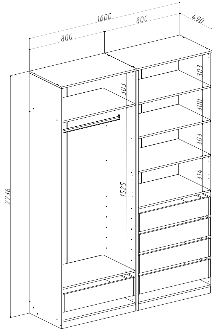
Ларго Вариант №7 (без фасадов) (ШхВхГ) 1600х2236х490 мм
