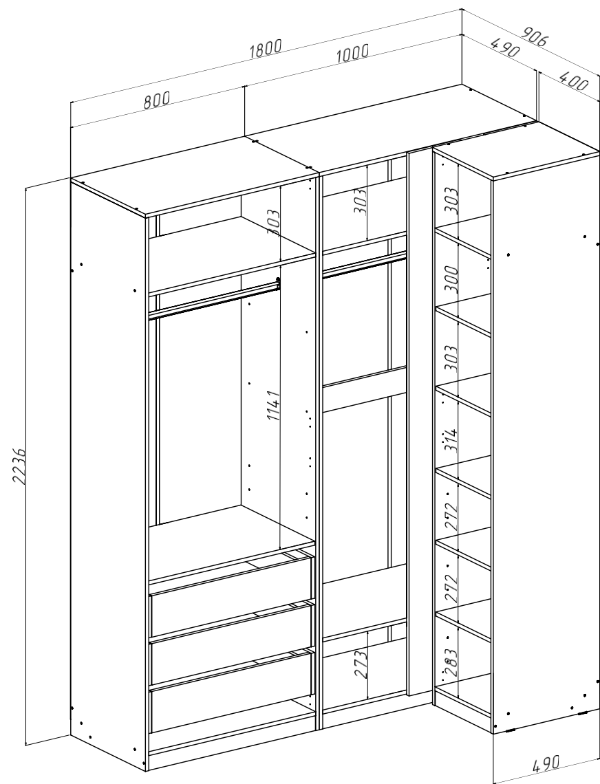
Ларго Вариант №11 (без фасадов) (ШхВхГ) 1800х2236х906 мм
