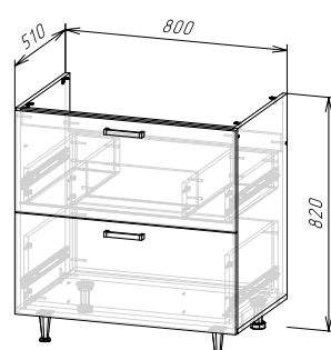
Корпус: ШНМ2ЯГ800(490) (ШхВхГ) 800х820х510 мм Фасад: ФАСАД ШНМ2ЯГ800
