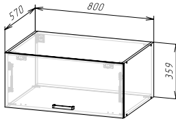
Корпус: ШВГА800/360 (ШхВхГ) 800x359x570 мм Фасад: ФАСАД ШВГ800/360 / ШВГА 800/360
