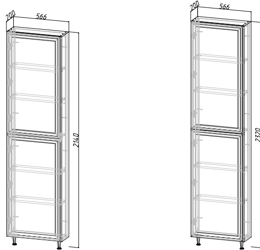
Корпус: ТР-П200 (ШхВхГ) 200х2140х566 мм Фасад: РАМКА AGT ТР-П200
