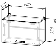
Корпус: ШВГ600/360 / ШВГС600/360 (ШхВхГ) 600х359х300 мм Фасад: ФАСАД ШВГ600/360 / ШВГА 600/360
