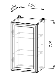
Корпус: ШВ400/ШВС400 (ШхВхГ) 400x718x300 мм Фасад: ФАСАД (РАМКА АГТ ШВС400)
