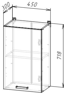
Корпус: ШВ450/ШВС450 (ШхВхГ) 450х718х300 мм Фасад: ФАСАД ШВ450/ШН450
