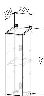
Корпус: ШВ200 (ШхВхГ) 200х718х300 мм Фасад: ФАСАД ШВ200/ШН200
