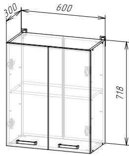
Корпус: ШВ600/ШВС600/ ШВ1Д600/ШВС1Д600 (ШхВхГ) 600х718х300 мм Фасад: ФАСАД ШВ600/ШН600/ШНМ600
