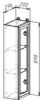
Корпус: ШВТД200/900 (ШхВхГ) 200x898x300 мм Фасад: ФАСАД ШВТД200/900
