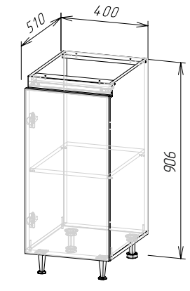
Корпус: ШН400(Техно-6) (ШхВхГ) 400х906х510 мм Фасад: ФАСАД ТЕХНО-6 ШН400
