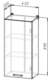
Корпус: ШВ450/ШВС450 (ШхВхГ) 450х898х300 мм Фасад: ФАСАД ШВ450/900
