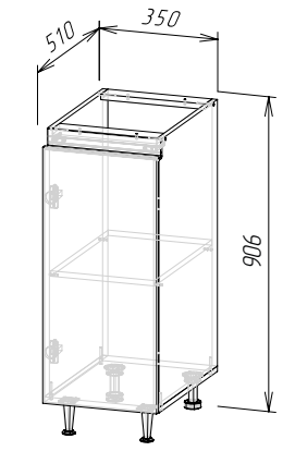
Корпус: ШН350/ШН450(Техно-6) (ШхВхГ) 350х906х510 мм Фасад: ФАСАД ТЕХНО-6 ШН350
