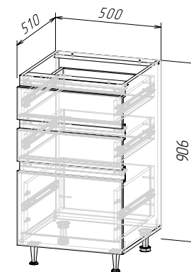
Корпус: ШНЗЯГ500(Техно-6) (ШхВхГ) 500х906х510 мм Фасад: ФАСАД ТЕХНО-6 ШНЗЯГ500
