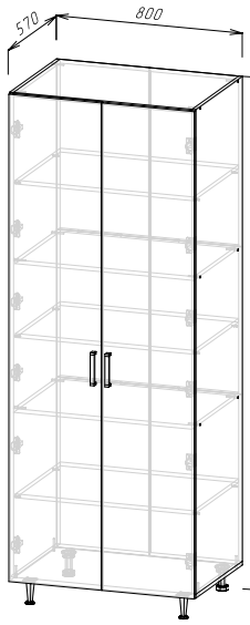
Корпус: ШП800/ШПС800/ ШП800-1 (ШхВхГ) 800x2140x570 мм Фасад: ФАСАД ШП800-1
