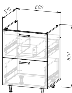
Корпус: ШНМ2ЯГ600(490) (ШхВхГ) 600х820х510 мм Фасад: ФАСАД ШНМ2ЯГ600
