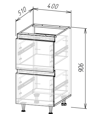
Корпус: ШН2ЯГ400(Техно-6) (ШхВхГ) 400х906х510 мм Фасад: ФАСАД ТЕХНО-6 ШН2ЯГ400
