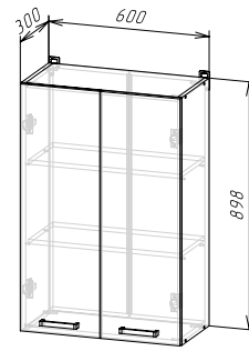
Корпус: ШВ600/900 / ШВС600/900/ ШВ1Д600/900 / ШВС1Д600/900 (ШхВхГ) 600х898х300 мм Фасад: ФАСАД ШВ600/900
