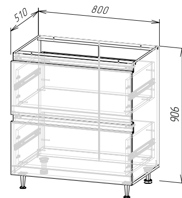
Корпус: ШНЗЯГ800(Техно-6) (ШхВхГ) 800х906х510 мм Фасад: ФАСАД ТЕХНО-6 ШНЗЯГ800/ ШНМЗЯГ800
