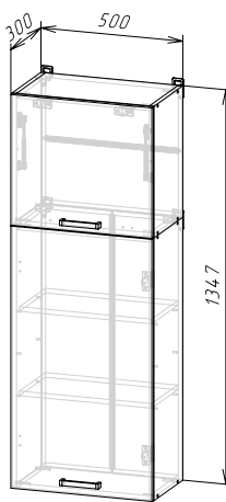
Корпус: ШВ500/1350 (ШxBxГ) 500x1347x300 мм Фасад: ФАСАД ШВ500/1350
