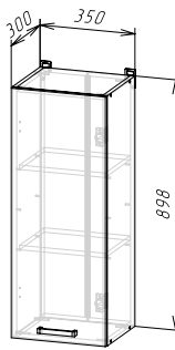
Корпус: ШВ350/900 (ШхВхГ) 350х898х300 мм Фасад: ФАСАД ШВ350/900
