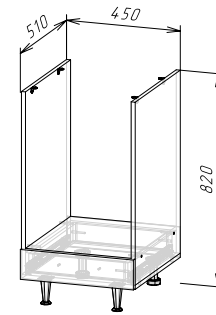
Корпус: ШНВТ450(490) (ШхВхГ) 450х820х510 мм Фасад: ФАСАД ШНВТ450
