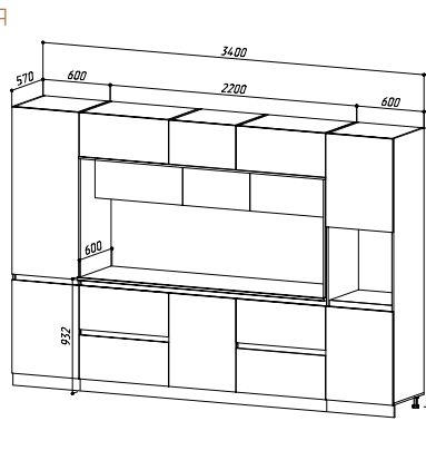
ЦЕНТРАЛЬНАЯ СЕКЦИЯ 2200+ПЕНАЛ+ПЕНАЛ ДЛЯ ВСТРАИВАЕМОЙ БЫТОВОЙ ТЕХНИКИ КОМПОНОВКА #3 (ШхВхГ) 3400х2268х600 мм Ручки: профиль GOLA (алюминий) Цоколь: входит в комплект
