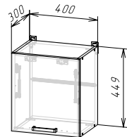
Корпус: ШВГ400/450 (ШхВхГ) 400x449x300 мм Фасад: ФАСАД ШВГ400/450
