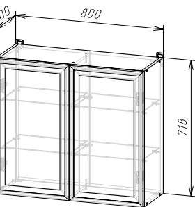
Корпус: ШВСП 800 НИКОЛЬ (ШхВхГ) 800x718x300 мм Фасад: ФАСАД (РАМКА АГТ ШВС800)
