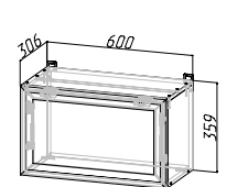
Корпус: ШВГ-П600/360 (ШхВхГ) 600х359х306 мм Фасад: РАМКА AGT ШВГ/ШВГА 600/360
