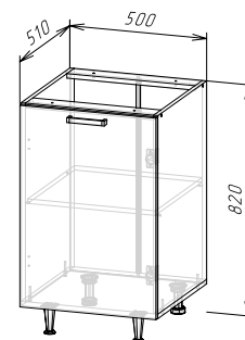
Корпус: ШН500(490) (ШхВхГ) 500х820х510 мм Фасад: ФАСАД ШВ500/ШН500/ШНМ500
