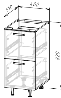
Корпус: ШН2ЯГ400(490) (ШхВхГ) 400х820х510 мм Фасад: ФАСАД ШН2ЯГ400
