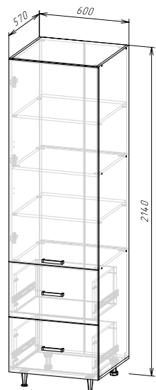
Корпус: ШП2Я600/ШП2Я600-1/ ШП2Я600-2 (ШхВхГ) 600x2140x570 мм Фасад: ФАСАД ШП2Я600-2
