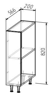
Корпус: ТР 820 (БЕЗ СТОЛЕШНИЦЫ) (ШхВхГ) 200x820x566 мм
