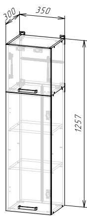
Корпус: ШВ350/1260 (ШхВхГ) 350x1257x300 мм Фасад: ФАСАД ШВ350/1260
