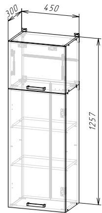
Корпус: ШВ450/1260 (ШxBxГ) 450x1257x300 мм Фасад: ФАСАД ШВ450/1260
