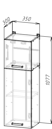
Корпус: ШВ350/1080 (ШхВхГ) 350x1077x300 мм Фасад: ФАСАД ШВ350/1080
