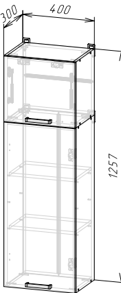
Корпус: ШВ400/1260 (ШхВхГ) 400x1257x300 мм Фасад: ФАСАД ШВ400/1260
