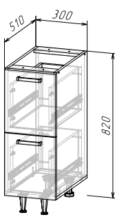
Корпус: ШН2ЯГ300(490) (ШхВхГ) 300х820х510 мм Фасад: ФАСАД ШН2ЯГ300
