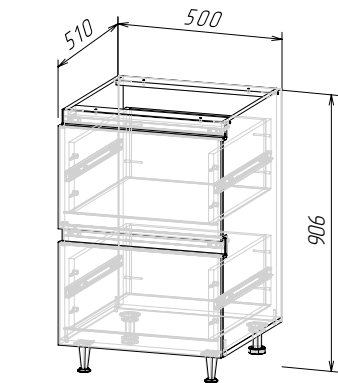
Корпус: ШН2ЯГ500(Техно-6) (ШхВхГ) 500х906х510 мм Фасад: ЛДСП ФАСАД ТЕХНО-6 ШН2ЯГ500
