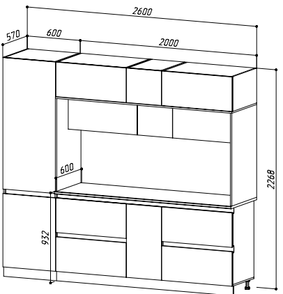
ЦЕНТРАЛЬНАЯ СЕКЦИЯ 2000+ПЕНАЛ КОМПОНОВКА #1 (ШхВхГ) 2600х2268х600 мм Ручки: профиль GOLA (алюминий) Цоколь: входит в комплект
