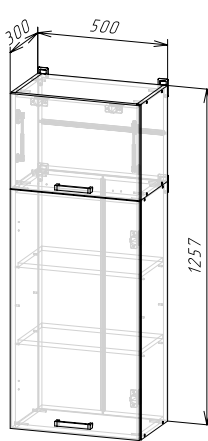
Корпус: ШВ500/1260 (ШxBxГ) 500x1257x300 мм Фасад: ФАСАД ШВ500/1260
