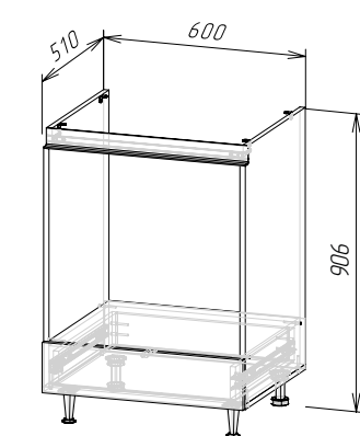
Корпус: ШНБТ600(Техно-6) (ШхВхГ) 600х906х510 мм Фасад: ФАСАД ТЕХНО-6 ШНБТ600
