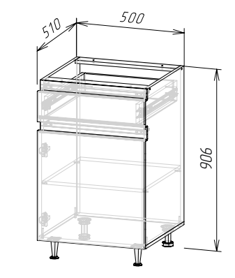
Корпус: ШН1Я500(Техно-6) (ШхВхГ) 500х906х510 мм Фасад: ФАСАД ТЕХНО-6 ШН1Я500
