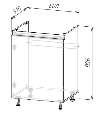
Корпус: ШНМ1Д600(Техно-6) (ШхВхГ) 600х906х510 мм Фасад: ФАСАД ТЕХНО-6 ШН1Д600/ШНМ1Д600
