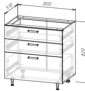
Корпус: ШНЗЯ800(490) (ШхВхГ) 800х820х510 мм Фасад: ФАСАД ШНЗЯ800
