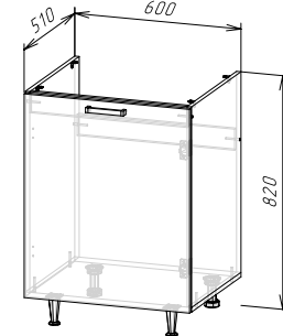
Корпус: ШНМ600/ШНМ1Д600(490) (ШхВхГ) 600х820х510 мм Фасад: ФАСАД ШВ1Д600/ШН1Д600/ШНМ1Д600
