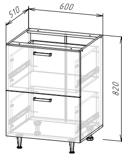
Корпус: ШН2ЯГ600(490) (ШхВхГ) 600х820х510 мм Фасад: ФАСАД ШН2ЯГ600
