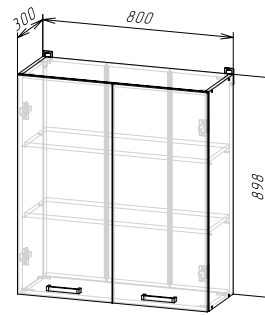
Корпус: ШВ800/900/ШВС800/900 (ШхВхГ) 800х898х300 мм Фасад: ФАСАД ШВ800/900
