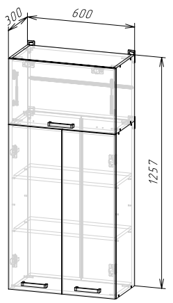
Корпус: ШВ600/1260 (ШxBxГ) 600x1257x300 мм Фасад: ФАСАД ШВ600/1260
