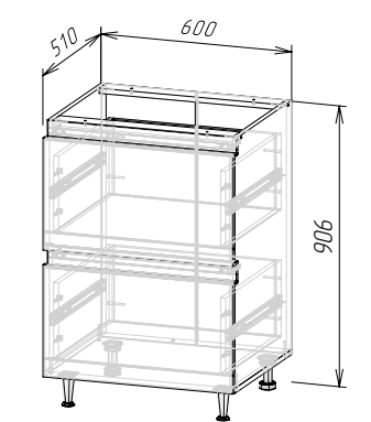
Корпус: ШН2ЯГ600(Техно-6) (ШхВхГ) 600х906х510 мм Фасад: ФАСАД ТЕХНО-6 ШН2ЯГ600/ ШНМ2ЯГ600
