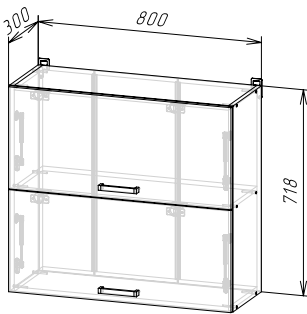
Корпус: ШВГ800/ШВГС800 (ШхВхГ) 800x718x300 мм Фасад: ФАСАД ШВГ800
