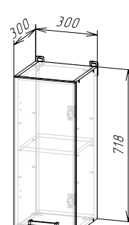
Корпус: ШВ300/ШВС300 (ШхВхГ) 300х718х300 мм Фасад: ФАСАД ШВ300/ШН300
