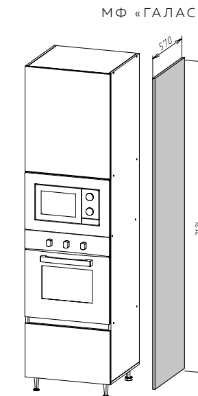
ФАСАД ТЕХНО-6 БФП (2124х570) (ШхВхГ) 570х2124х16 мм
