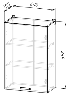
Корпус: ШВ600/900 / ШВС600/900/ ШВ1Д600/900 / ШВС1Д600/900 (ШхВхГ) 600х898х300 мм Фасад: ФАСАД ШВ1Д600/900
