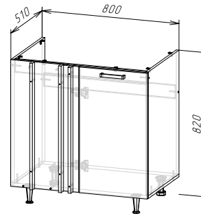
Корпус: ШНУ1000(490) (ШхВхГ) 800х820х510 мм Фасад: ФАСАД ШНУ1000
