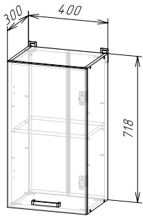
Корпус: ШВ400/ШВС400 (ШхВхГ) 400х718х300 мм Фасад: ФАСАД ШВ400/ШН400
