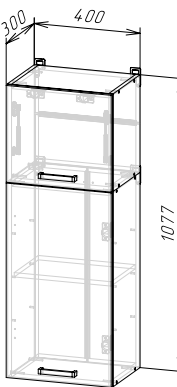
Корпус: ШВ400/1080 (ШхВхГ) 400x1077x300 мм Фасад: ФАСАД ШВ400/1080
