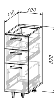
Корпус: ШНЗЯ300(490) (ШхВхГ) 300х820х510 мм Фасад: ФАСАД ШНЗЯ300
