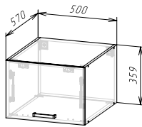
Корпус: ШВГА500/360 (ШхВхГ) 500x359x570 мм Фасад: ФАСАД ШВГ500/360 / ШВГА 500/360
