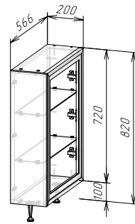
Корпус: ШНТД200 (ШхВхГ) 200х820х566 мм Фасад: ФАСАД ШВТД200/ ШНТД200
