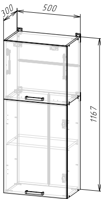
Корпус: ШВ500/1170 (ШxBxГ) 500x1167x300 мм Фасад: ФАСАД ШВ500/1170
