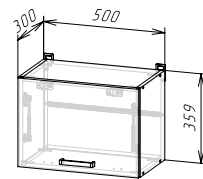
Корпус: ШВГ500/360 / ШВГС500/360 (ШхВхГ) 500х359х300 мм Фасад: ФАСАД ШВГ500/360 / ШВГА 500/360
