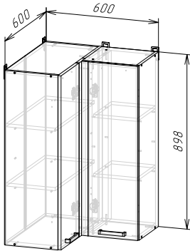
Корпус: ШВУП600/900 (ШхВхГ) 600x898x600 мм Фасад: ФАСАД ШВУП600/900
