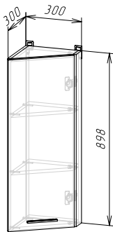
Корпус: ШВТД300/900 (ШхВхГ) 300x898x300 мм Фасад: ФАСАД ШВТД300/900
