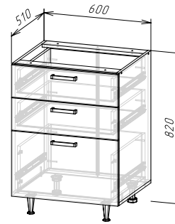
Корпус: ШНЗЯ600(490) (ШхВхГ) 600х820х510 мм Фасад: ФАСАД ШНЗЯ600
