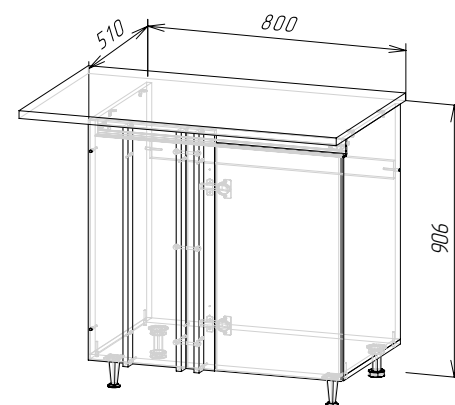
Корпус: ШНУ1000(Техно-6) (ШхВхГ) 800х906х510 мм Фасад: ФАСАД ТЕХНО-6 ШНУ1000
