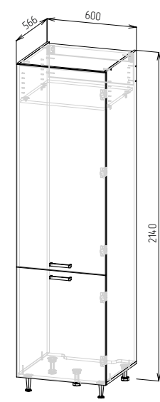
Корпус: ШПХ600 (ШхВхГ) 600x2140x566 мм Фасад: ФАСАД ШП600-2/ШХ
