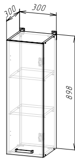
Корпус: ШВ300/900 / ШВС300/900 (ШхВхГ) 300х898х300 мм Фасад: ФАСАД ШВ300/900
