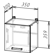
Корпус: ШВГ350/360 (ШхВхГ) 350х359х300 мм Фасад: ФАСАД ШВГ350/360 / ШВГА 350/360
