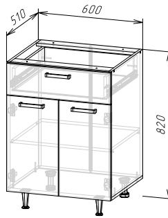
Корпус: ШН1Я600/ШН1Д1Я600(490) (ШхВхГ) 600х820х510 мм Фасад: ФАСАД ШН1Я600
