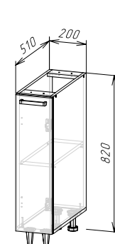
Корпус: ШН200(490) (ШхВхГ) 200х820х510 мм Фасад: ФАСАД ШВ200/ШН200
