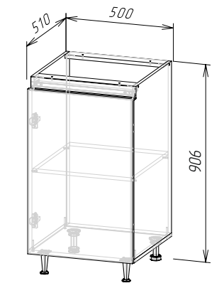
Корпус: ШН500(Техно-6) (ШхВхГ) 500х906х510 мм Фасад: ФАСАД ТЕХНО-6 ШН500/ШНМ500
