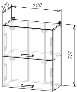
Корпус: ШВГ600/ШВГС600 (ШхВхГ) 600x718x300 мм Фасад: ФАСАД ШВГ600
