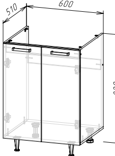
Корпус: ШНМ600/ШНМ1Д600(490) (ШхВхГ) 600х820х510 мм Фасад: ФАСАД ШВ600/ШН600/ШНМ600
