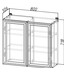
Корпус: ШВСП-П800 (ШхВхГ) 800х718х306 мм Фасад: РАМКА AGT ШВ800
