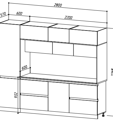
ЦЕНТРАЛЬНАЯ СЕКЦИЯ 2200+ПЕНАЛ КОМПОНОВКА #1 (ШхВхГ) 2800х2268х600 мм Ручки: профиль GOLA (алюминий) Цоколь: входит в комплект
