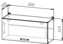
Корпус: ШВГ800/360 / ШВГС800/360 (ШхВхГ) 800х359х300 мм Фасад: ФАСАД ШВГ800/360 / ШВГА 800/360
