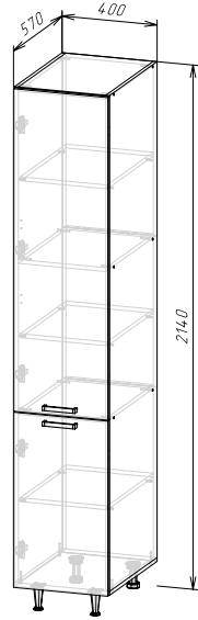
Корпус: ШП400/ШП400-1 (ШхВхГ) 400x2140x570 мм Фасад: ФАСАД ШП400-1
