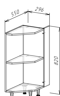
Корпус: ШНТ300 (ШхВхГ) 296х820х550 мм
