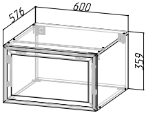
Корпус: ШВГА-П600/360 (ШхВхГ) 600х359х576 мм Фасад: РАМКА AGT ШВГ/ШВГА 600/360
