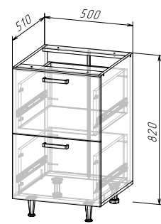
Корпус: ШН2ЯГ500(490) (ШхВхГ) 500х820х510 мм Фасад: ФАСАД ШН2ЯГ500
