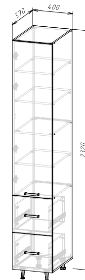
Корпус: ШПВ2Я400/ШПВ2Я400-1 (ШхВхГ) 400х2320х570 мм Фасад: ФАСАД ШПВ2Я400-1
