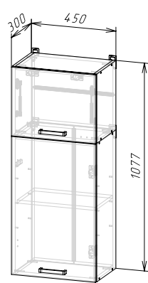
Корпус: ШВ450/1080 (ШxBxГ) 450x1077x300 мм Фасад: ФАСАД ШВ450/1080
