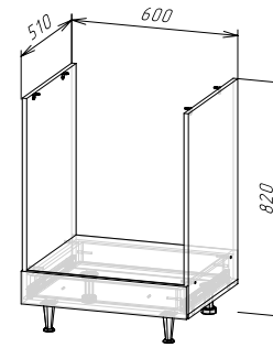
Корпус: ШНВТ600(490) (ШхВхГ) 600х820х510 мм Фасад: ФАСАД ШНВТ600
