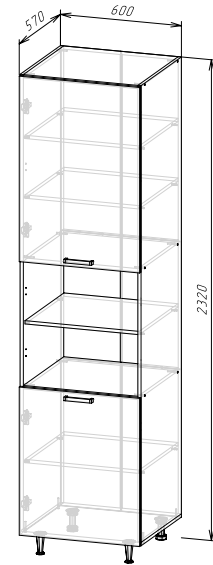
Корпус: ШПВ600/ШПВ600-1/ШПВ600-2 (ШхВхГ) 600х2320х570 мм Фасад: ФАСАД ШПВ600
