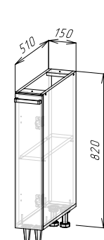
Корпус: ШН150(490) (ШхВхГ) 150х820х510 мм Фасад: ФАСАД ШВ150/ШН150
