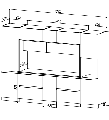
ЦЕНТРАЛЬНАЯ СЕКЦИЯ 2050 (С МЕСТОМ ПОД МП)+ПЕНАЛ+ПЕНАЛ ДЛЯ ВСТРАИВАЕМОЙ БЫТОВОЙ ТЕХНИКИ КОМПОНОВКА #3 (ШхВхГ) 3250х2268х600 мм место под МП (ШхВхГ) 450х849х533 мм Ручки: профиль GOLA (алюминий) Цоколь: входит в комплект
