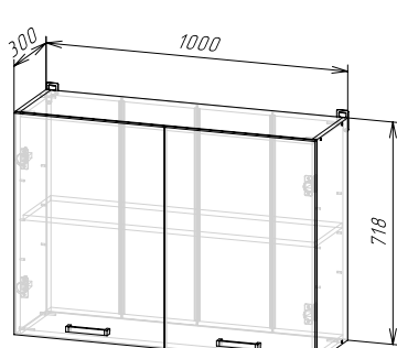
Корпус: ШВ1000/ШВС1000 (ШхВхГ) 1000х718х300 мм Фасад: ФАСАД ШВ1000
