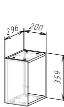
Корпус: ШВТ200/360 (ШхВхГ) 200x359x300 мм Фасад: ФАСАД ШВТ200/360
