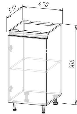
Корпус: ШН350/ШН450(Техно-6) (ШхВхГ) 450х906х510 мм Фасад: ФАСАД ТЕХНО-6 ШН450
