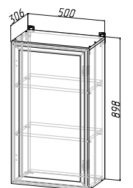
Корпус: ШВ-П500/900 (ШхВхГ) 500х898х306 мм Фасад: РАМКА AGT ШВ500/900
