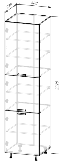
Корпус: ШПВ600/ШПВ600-1/ШПВ600-2 (ШхВхГ) 600х2320х570 мм Фасад: ФАСАД ШПВ600-1
