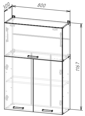
Корпус: ШВ800/1170 (ШxBxГ) 800x1167x300 мм Фасад: ФАСАД ШВ800/1170
