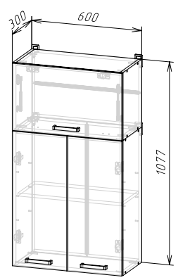
Корпус: ШВ600/1080 (ШxBxГ) 600x1077x300 мм Фасад: ФАСАД ШВ600/1080
