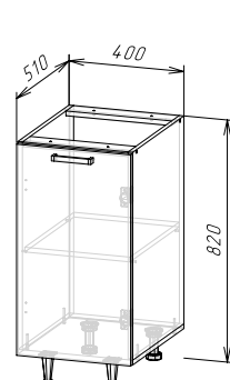
Корпус: ШН400(490) (ШхВхГ) 400х820х510 мм Фасад: ФАСАД ШВ400/ШН400
