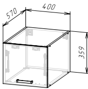
Корпус: ШВГА400/360 (ШхВхГ) 400x359x570 мм Фасад: ФАСАД ШВГ400/360 / ШВГА 400/360
