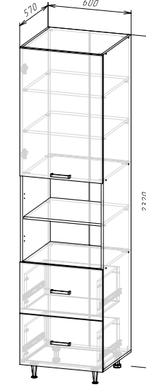
Корпус: ШПВ2Я600/ШПВ2Я600-1/ ШПВ2Я600-2 (ШхВхГ) 600х2320х570 мм Фасад: ФАСАД ШПВ2Я600
