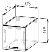
Корпус: ШВГА350/360 (ШхВхГ) 350x359x570 мм Фасад: ФАСАД ШВГ350/360 / ШВГА 350/360
