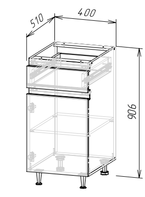
Корпус: ШН1Я400(Техно-6) (ШхВхГ) 400х906х510 мм Фасад: ФАСАД ТЕХНО-6 ШН1Я400
