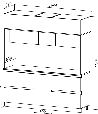
ЦЕНТРАЛЬНАЯ СЕКЦИЯ 2050 (С МЕСТОМ ПОД МП) (ШхВхГ) 2050х2268х600 мм место под МП (ШхВхГ) 450х849х533 мм Ручки: профиль GOLA (алюминий) Цоколь: входит в комплект
