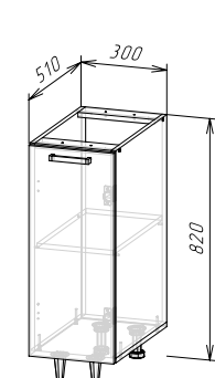
Корпус: ШН300(490) (ШхВхГ) 300х820х510 мм Фасад: ФАСАД ШВ300/ШН300
