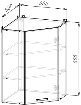
Корпус: ШВУ600/900 / ШВУС600/900 (ШхВхГ) 600x898x600 мм Фасад: ФАСАД ШВУ600/900
