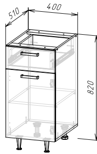
Корпус: ШН1Я400(490) (ШхВхГ) 400х820х510 мм Фасад: ФАСАД ШН1Я400
