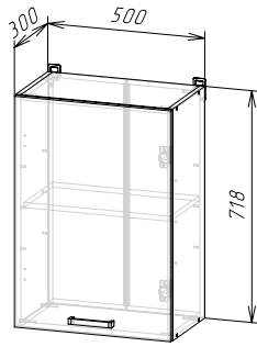
Корпус: ШВ500/ШВС500 (ШхВхГ) 500х718х300 мм Фасад: ФАСАД ШВ500/ШН500/ШНМ500
