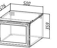
Корпус: ШВГА-П500/360 (ШхВхГ) 500х359х576 мм Фасад: РАМКА AGT ШВГ/ШВГА 500/360
