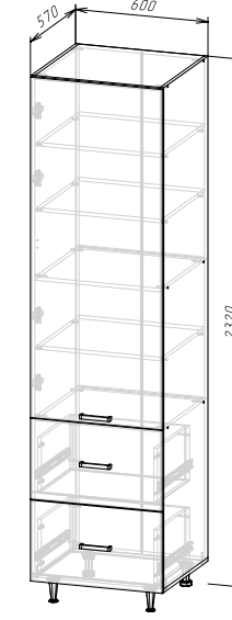
Корпус: ШПВ2Я600/ШПВ2Я600-1/ ШПВ2Я600-2 (ШхВхГ) 600х2320х570 мм Фасад: ФАСАД ШПВ2Я600-2
