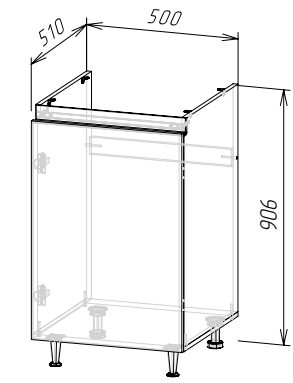
Корпус: ШНМ500(Техно-6) (ШхВхГ) 500х906х510 мм Фасад: ФАСАД ТЕХНО-6 ШН500/ШНМ500
