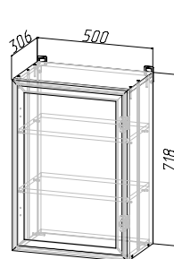
Корпус: ШВ-П500 (ШхВхГ) 500х718х306 мм Фасад: РАМКА AGT ШВ500
