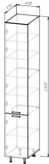
Корпус: ШПВ400/ШПВ400-1 (ШхВхГ) 400х2320х570 мм Фасад: ФАСАД ШПВ400-1
