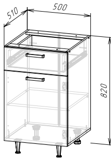
Корпус: ШН1Я500(490) (ШхВхГ) 500х820х510 мм Фасад: ФАСАД ШН1Я500
