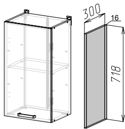
ЛДСП ФАСАД РИО NEW БФП (718x300) (ШхВхГ) 718x300x16 мм
