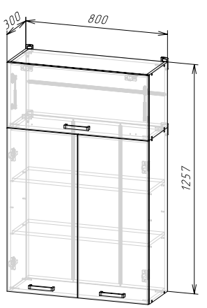
Корпус: ШВ800/1260 (ШxBxГ) 800x1257x300 мм Фасад: ФАСАД ШВ800/1260
