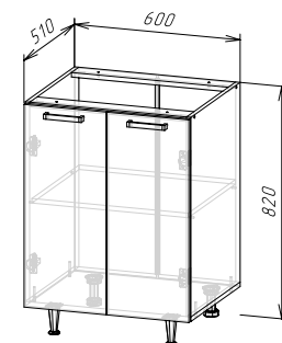
Корпус: ШН600/ШН1Д600(490) (ШхВхГ) 600х820х510 мм Фасад: ФАСАД ШВ600/ШН600/ШНМ600
