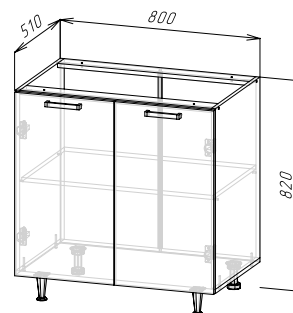
Корпус: ШН800(490) (ШхВхГ) 800х820х510 мм Фасад: ФАСАД ШВ800/ШН800/ШНМ800
