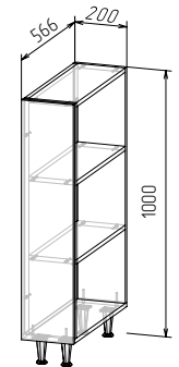
Корпус: ТР 1000 (ШхВхГ) 200x1000x566 мм
