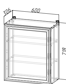
Корпус: ШВ1Д-П600 (ШхВхГ) 600х718х306 мм Фасад: РАМКА AGT ШВ1Д600
