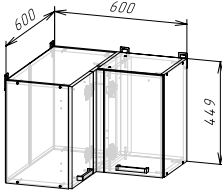
Корпус: ШВУП600/450 (ШхВхГ) 600x449x600 мм Фасад: ФАСАД ШВУП600/450
