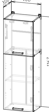
Корпус: ШВ400/1170 (ШхВхГ) 400x1167x300 мм Фасад: ФАСАД ШВ400/1170
