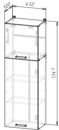
Корпус: ШВ450/1350 (ШxBxГ) 450x1347x300 мм Фасад: ФАСАД ШВ450/1350
