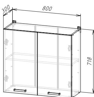
Корпус: ШВ800/ШВС800 (ШхВхГ) 800х718х300 мм Фасад: ФАСАД ШВ800/ШН800/ШНМ800
