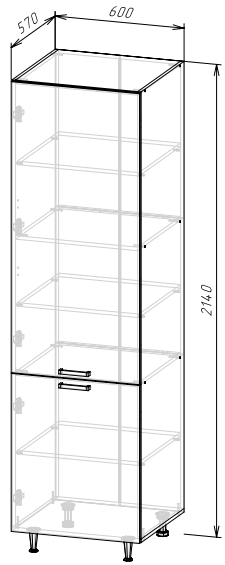
Корпус: ШП600/ШП600-1/ШП600-2 (ШхВхГ) 600x2140x570 мм Фасад: ФАСАД ШП600-2
