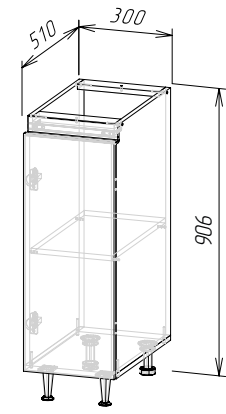
Корпус: ШН200/ШН300(Техно-6) (ШхВхГ) 300х906х510 мм Фасад: ФАСАД ТЕХНО-6 ШН300
