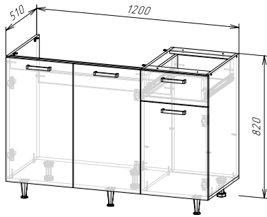
Корпус: ШН1Я1200(490) (ШхВхГ) 1200х820х510 мм Фасад: ФАСАД ШН1Я1200
