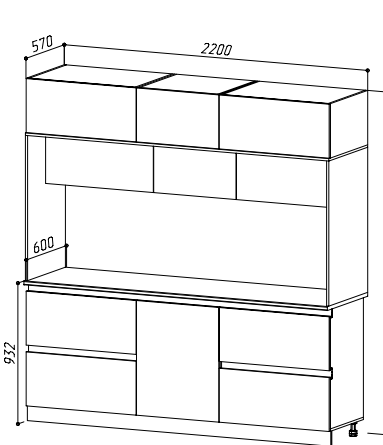
ЦЕНТРАЛЬНАЯ СЕКЦИЯ 2200 (ШхВхГ) 2200х2268х600 мм Ручки: профиль GOLA (алюминий) Цоколь: входит в комплект
