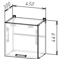
Корпус: ШВГ450/450 (ШхВхГ) 450x449x300 мм Фасад: ФАСАД ШВГ450/450 / ШВГА450/450
