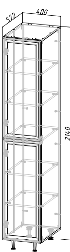
Корпус: ШП-П400 (ШхВхГ) 400х2140х572 мм Фасад: РАМКА AGT ШП-П400
