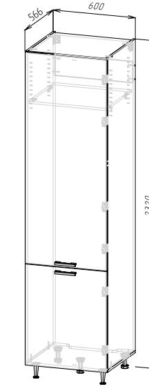
Корпус: ШПВХ600 (ШхВхГ) 600х2320х566 мм Фасад: ФАСАД ШПВ600-2/ШПВХ600
