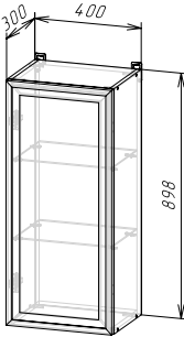
Корпус: ШВ400/900 / ШВС400/900 (ШхВхГ) 400x898x300 мм Фасад: ФАСАД (РАМКА АГТ ШВС400/900)
