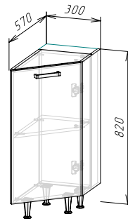
Корпус: ШНТД300 (ШхВхГ) 300х820х570 мм Фасад: ФАСАД ШНТД300
