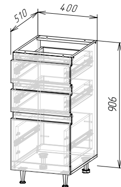
Корпус: ШНЗЯГ400(Техно-6) (ШхВхГ) 400х906х510 мм Фасад: ФАСАД ТЕХНО-6 ШНЗЯГ400
