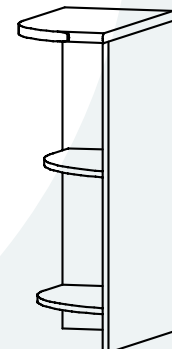
300 стол торц. 300×846×600*
