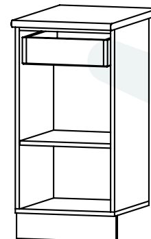
400стол с 1 ящ. 400×846×600*
