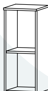
300 полка 300×736×300
