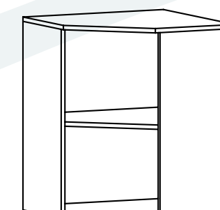
600/600 полка угловая 600×736×600
