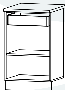
500стол с 1 ящ. 500×846×600*
