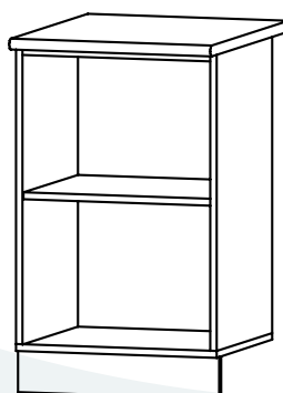
500 стол 500×846×600*
