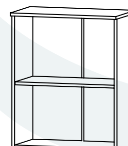
600 полка 600×736×300
