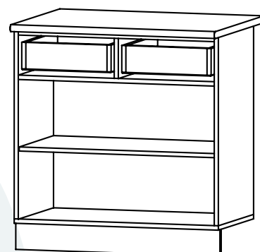
800 стол с 2 ящ. 800×846×600*
